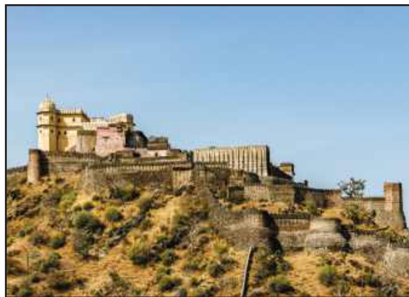
कुम्भलगढ़ : राजसमंद
